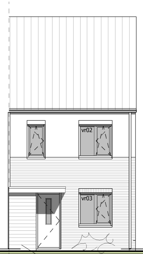
voorgevel 1 : 100
