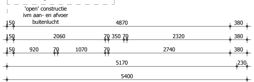
begane grond 1 : 50
