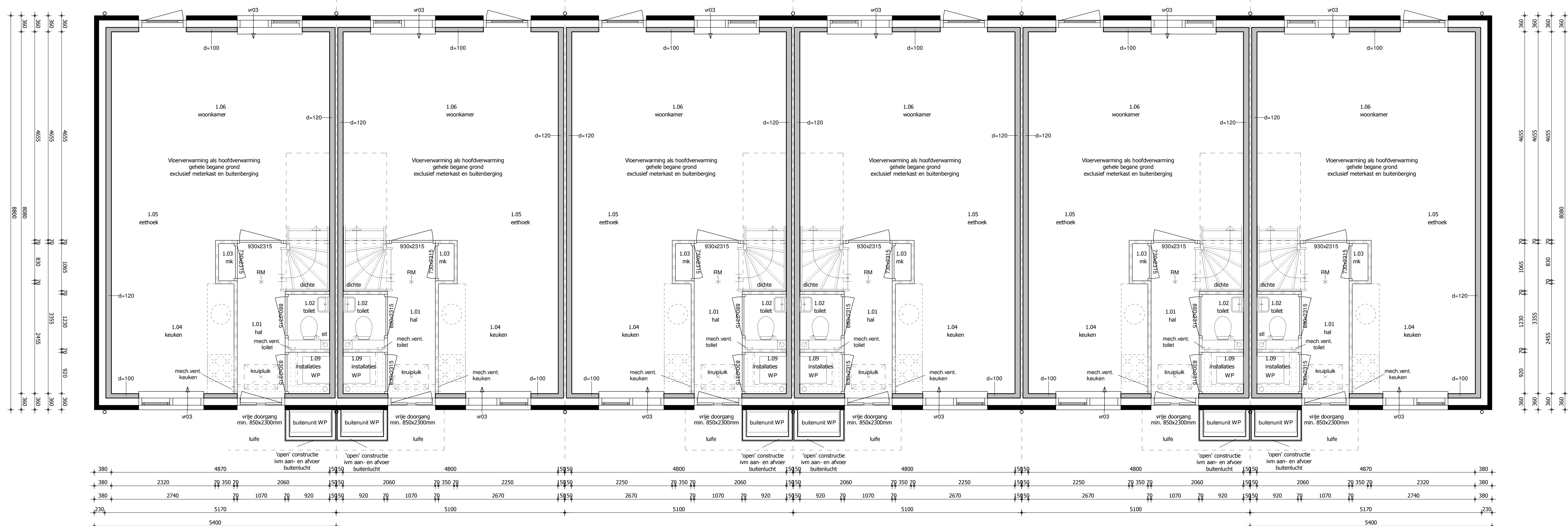
begane grond 1 : 50
